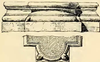
Fig. 378 — Base di una pilastretta dell'antica chiesa dei Santi Felice e Fortunato presso Vicenza (a. 985)
